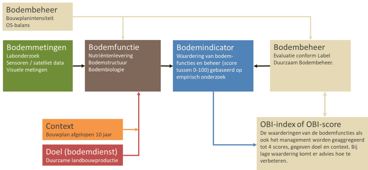
Figuur 1. Bodemwaarderingssystematiek zoals toegepast binnen de Open Bodemindex.
