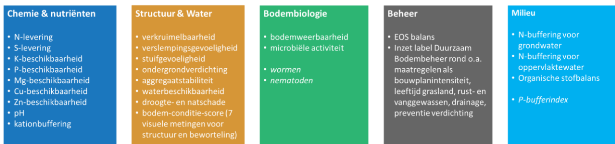
Figuur 2. Uitgewerkte bodemfuncties / indicatoren zoals deze zijn ingebed binnen de OBI, versie 0.11. De cursief weergegeven functies / indicatoren zijn kwalitatief beschreven, en daarom (nog) niet opgenomen in de berekening van de integrale bodemindex.
