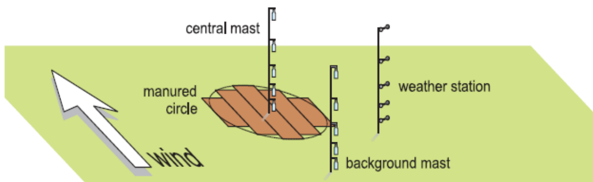
Figuur 2-3. De schematische weergave van een cirkelvormig veld voor de meting van NH 3 -emissie met behulp van de micro-meteorologische massabalansmethode, met masten met NH 3 -samplers op verschillende hoogtes in het midden van het perceel en aan de loefzijde van het perceel.
