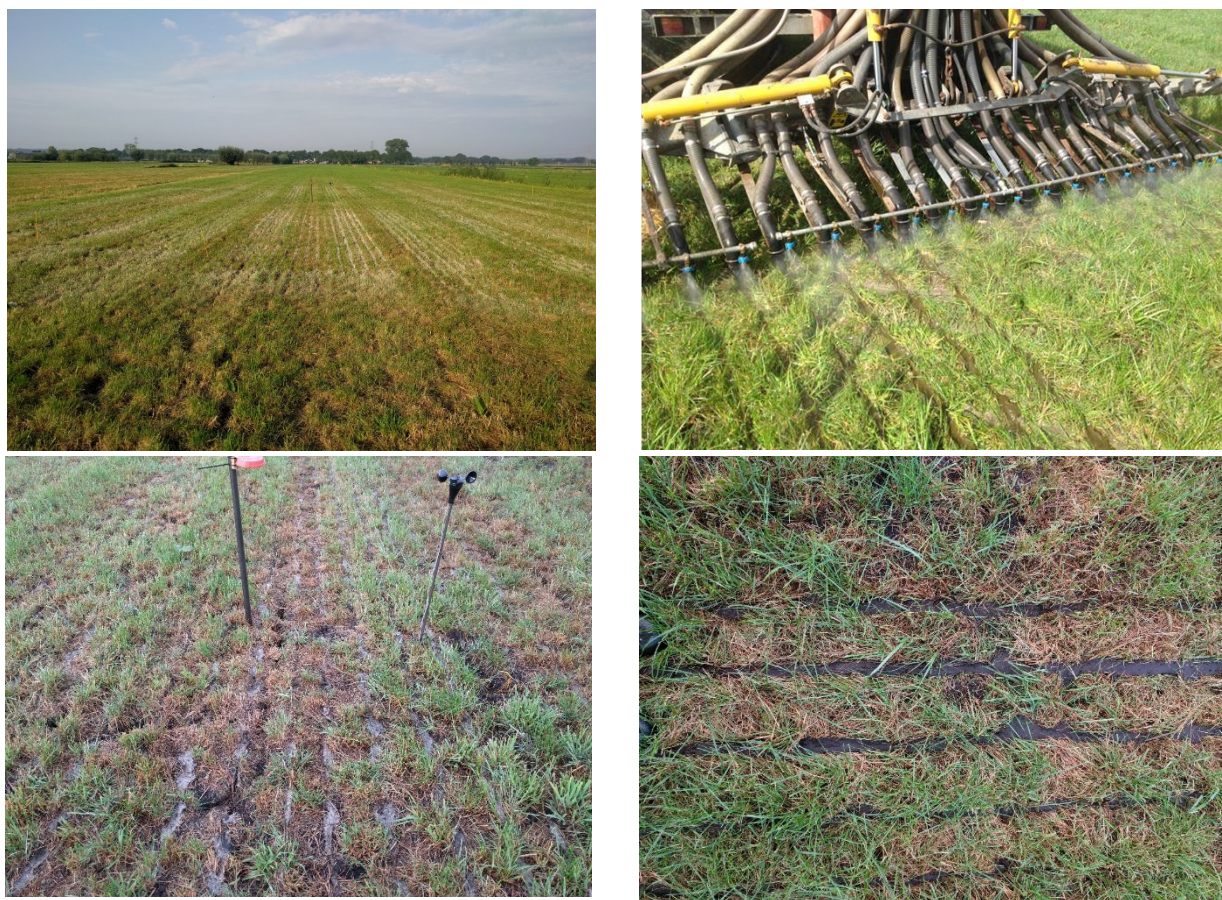
Figuur 4-2. Toediening van verdunde krijtsuspensie met mest via de Triple Spray in augustus 2019. De met Triple Spray toegediende mest is duidelijk herkenbaar aan de witte/grijze kleur in vergelijking tot zodenbemesting (plaatje rechtsonder). Op het plaatje linksonder is de meetpaal met afdekkapje te zien waaronder 3 passieve samplers zijn bevestigd. Op de sampler hoogte wordt ook de windsnelheid gemeten.
