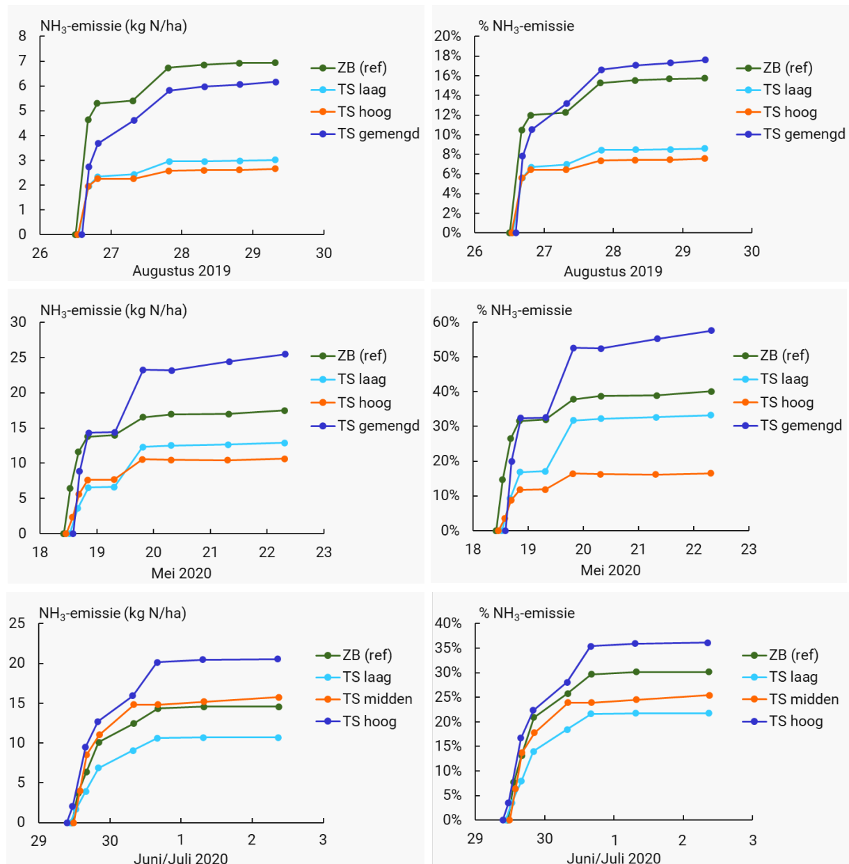
Figuur 4-5 De gemeten ammoniakemissie in augustus 2019, mei 2020 en juni 2020 met zodenbemesting (ZB) als referentietechniek ten opzichte van Triple Spray (TS) met een lage en hoge dosering krijtsuspensie en een variant waarbij de krijtsuspensie door de mest is gemengd. In juni 2020 is de behandeling TS gemengd vervangen door een sproeibehandeling met krijtsuspensie. In Tabel Y zijn de toegepaste dosering vermeld.
